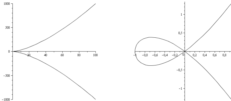
Abbildung 2.1: Neilsche Parabel (links) und Newtonscher Knoten.
