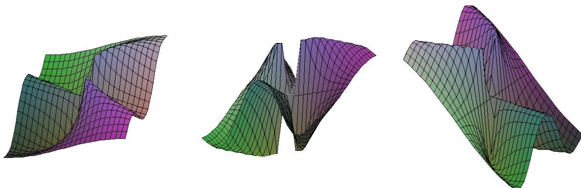
Abbildung 2.2: Die Funktion f(x, y) := \frac{xy^2}{x^2+y^4} für (x, y) \neq (0, 0) und f(0, 0) := 0 aus mehreren Perspektiven mittels MAPLE dargestellt.
