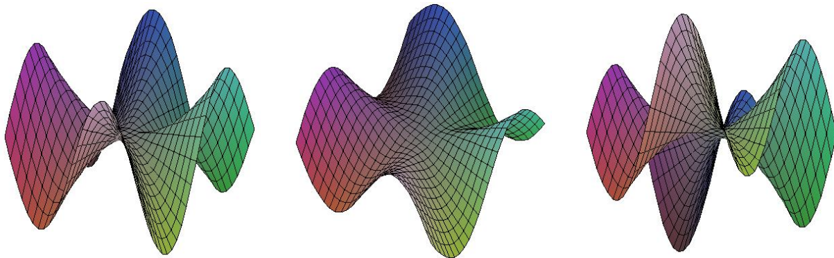
Abbildung 2.4: Die Funktion f(x, y) := \frac{x^3 y - x y^3}{x^2 + y^2} aus mehreren Perspektiven mittels MAPLE dargestellt.
