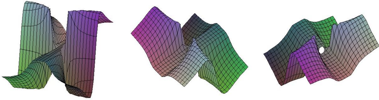
Abbildung 2.3: Die Funktion g(x, y) := \frac{2xe^{-1/y^2}}{x^2 + e^{-2/y^2}} für y \neq 0 und g(x, y) := 0 sonst aus mehreren Perspektiven mittels MAPLE dargestellt.
